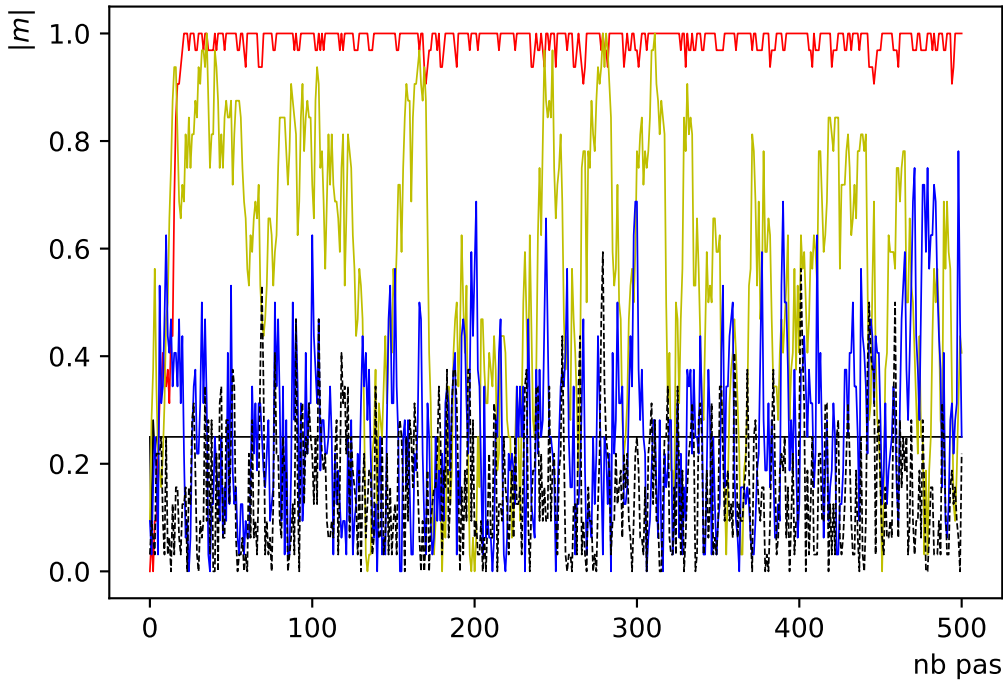
Evolution de l'aimantation sur 500 pas de Monte Carlo, N=8
